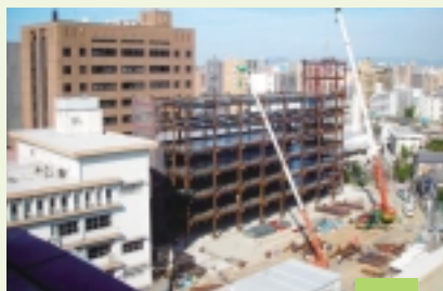
鉄骨組立中
